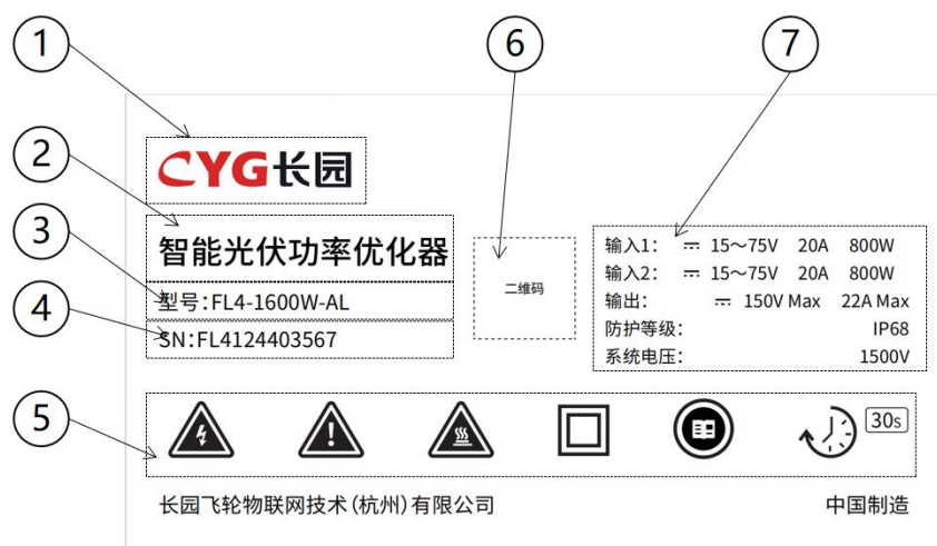
图 14 优化器铭牌
