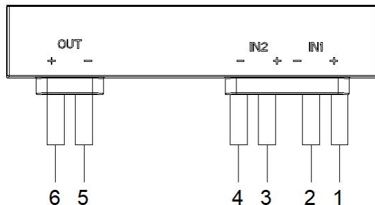
图4 产品接口说明
