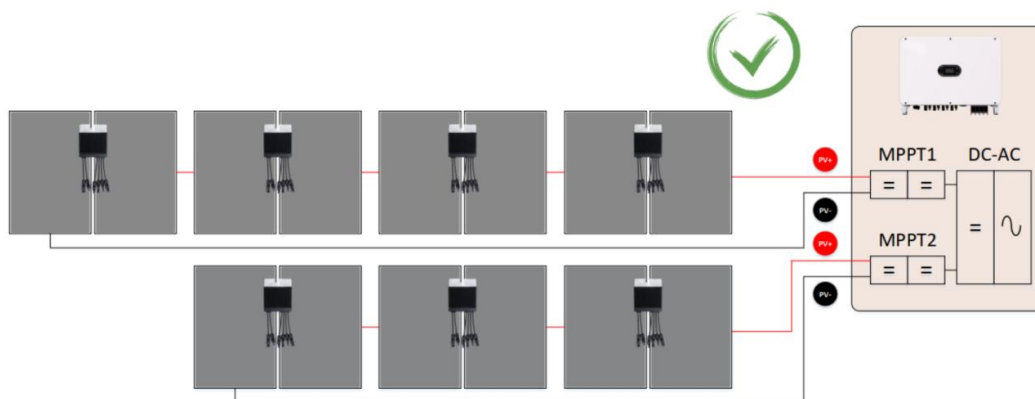
图 9 MPPT 之间若相互隔离，则可以分别配置优化器
