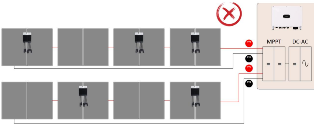
图 11 一路 MPPT 接入多路组串，不支持部分组件安装优化器
