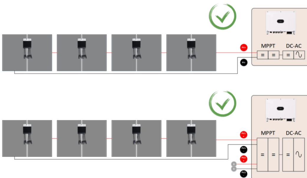
图 8 一路 MPPT 下安装一路组串，组件全部安装优化器
