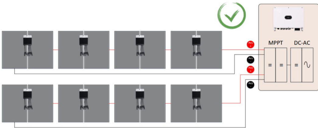
图 10 一路 MPPT 接入多路组串，组串中组件数量、型号需要完全一致，并且全部安装优化器
