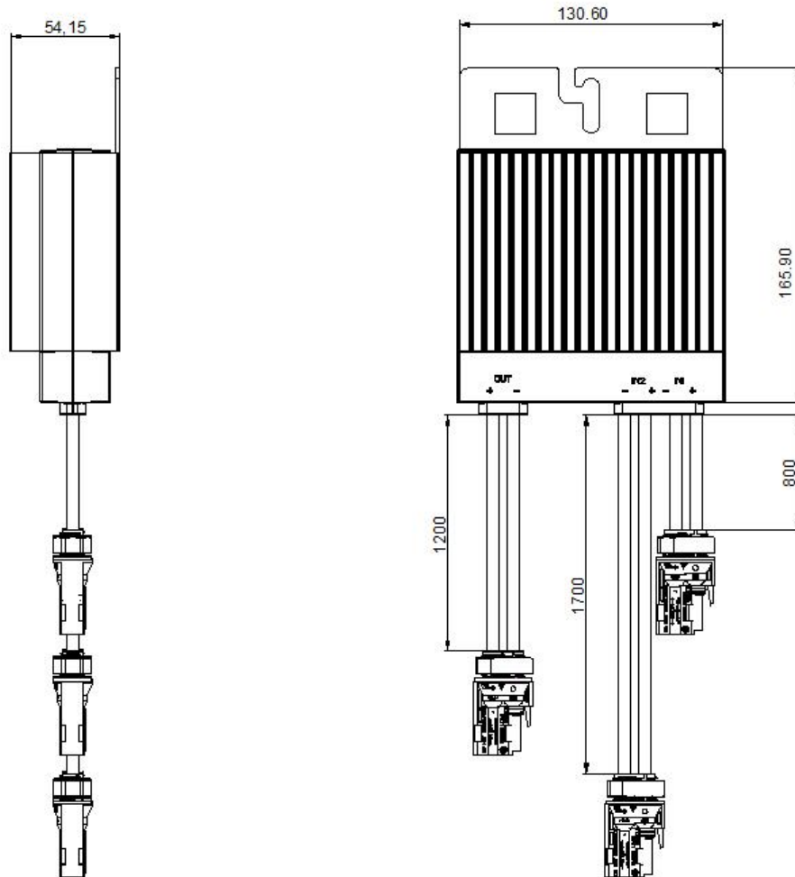
图 5 FL4-1600W-AL 产品尺寸
